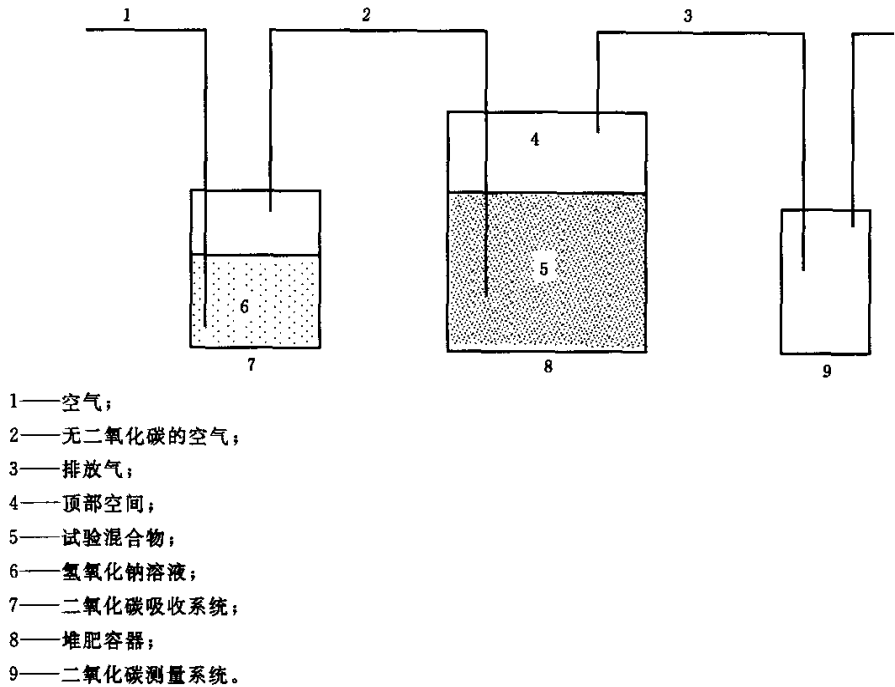
图 A.1 试验系统布置
